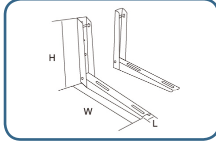
Teknik Çizim
